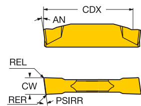
R123x2-CM
