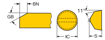
RPGX..S/T
