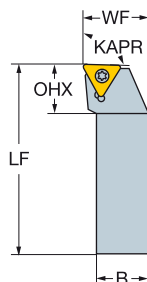
STFCR/L 91.0°
