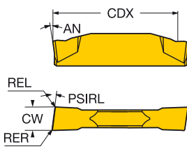
L123x2-CM
