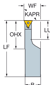
STFCR/L-A 90.0°
